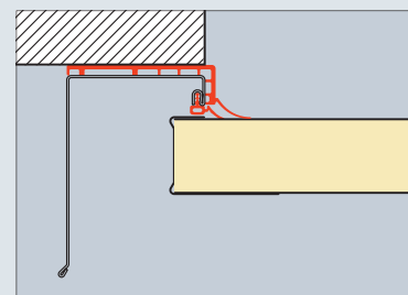
Boční ostění
